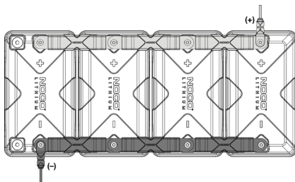
NLX 电池并联的正确配置。
