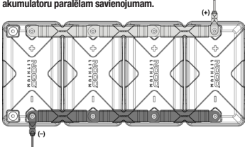
Pareiza akumulatoru konfigurācija NLX akumulatoru paralēlam savienojumam.
